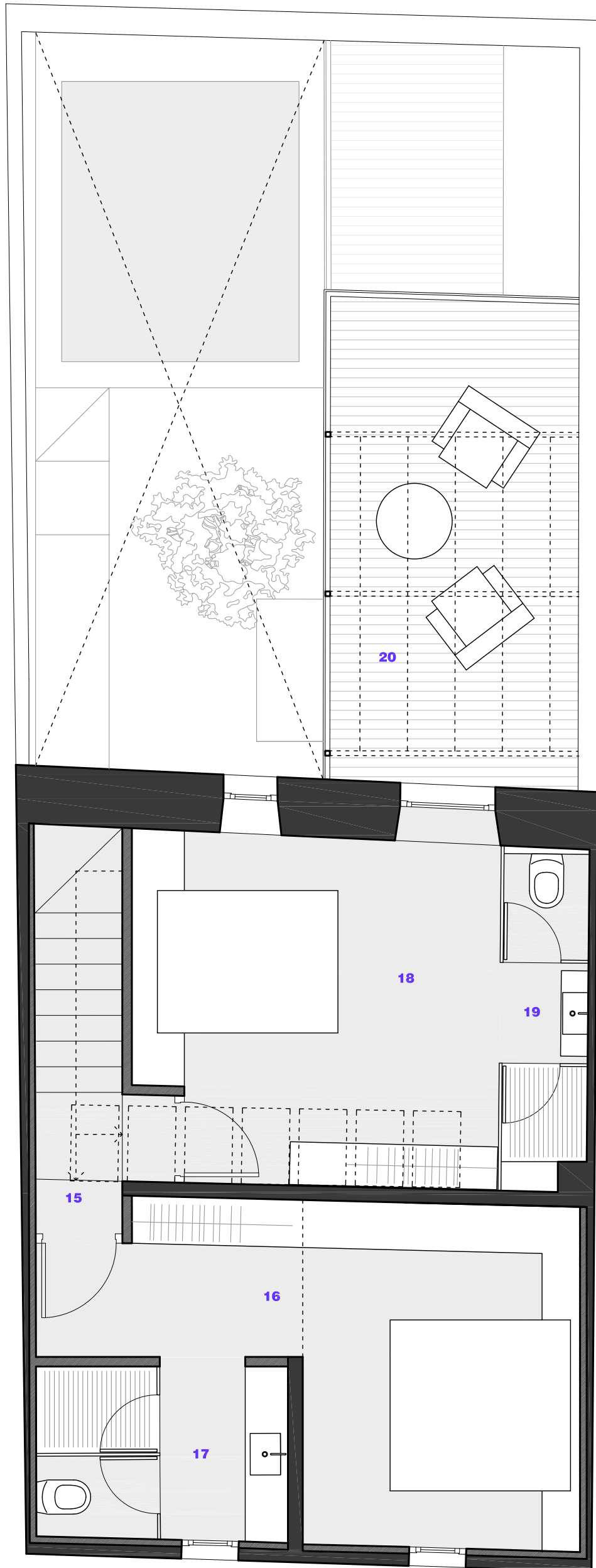
PLANTA PISO 2
