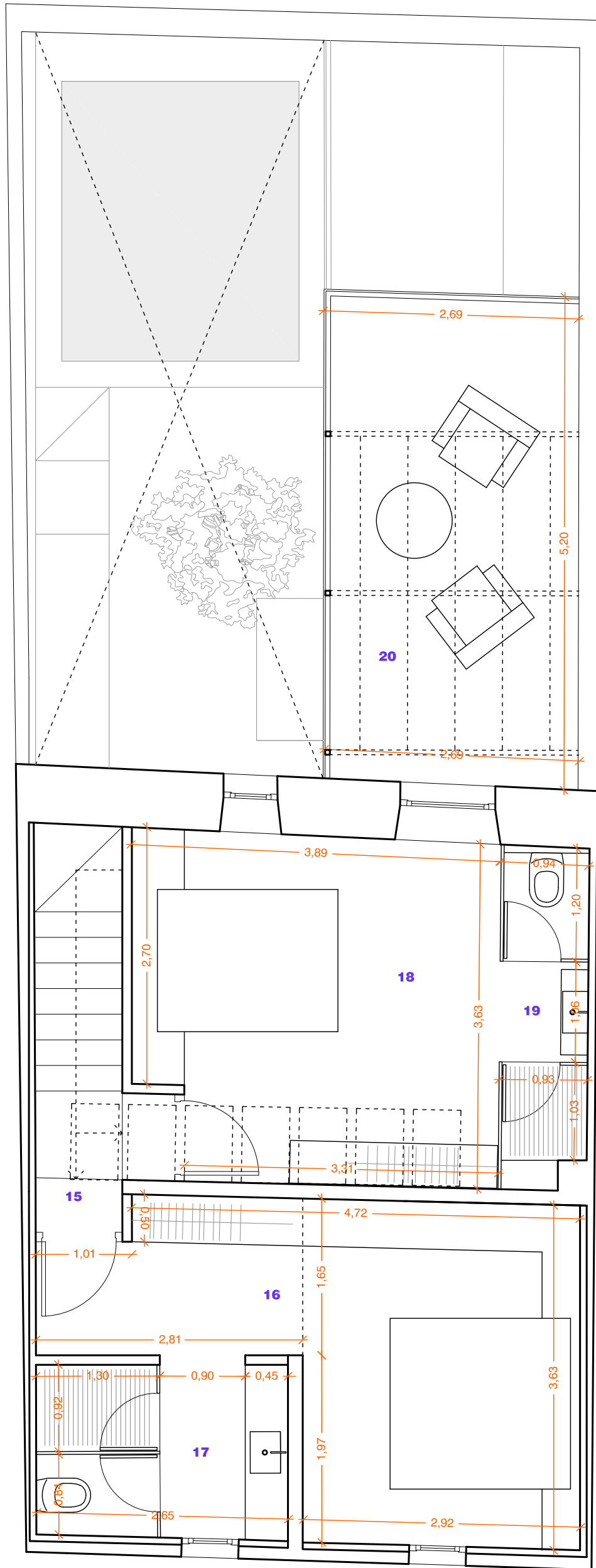
PLANTA PISO 2
