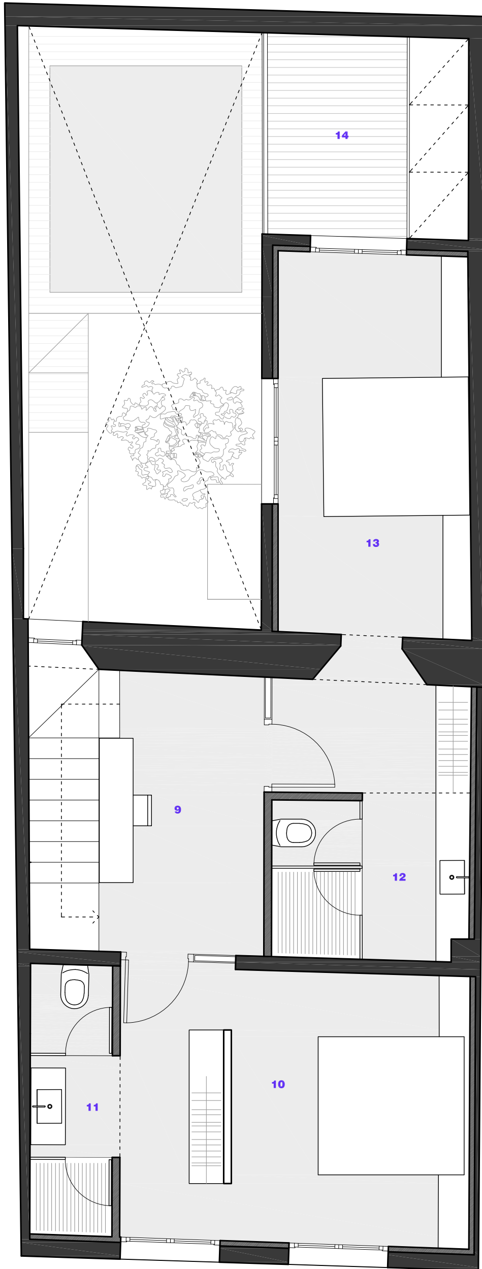
PLANTA PISO 1
